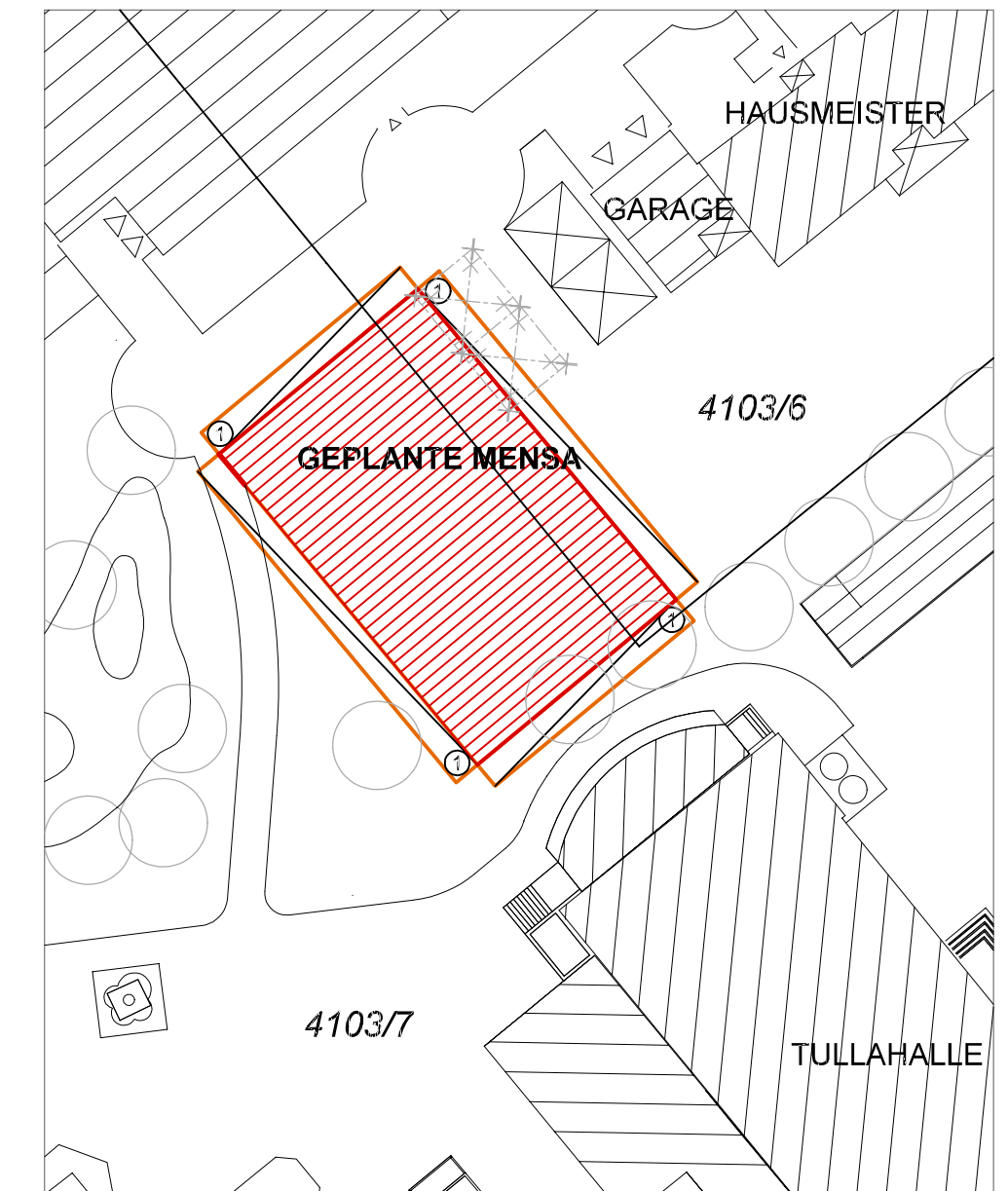
Abstandsflächen 1:500
